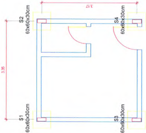
01 FORMAS FUNDAÇÃO Esc.: 1/50
