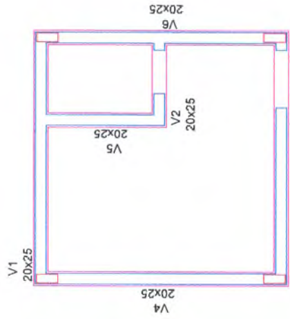
03 FORMAS BALDRAME Esc.: 1/50
