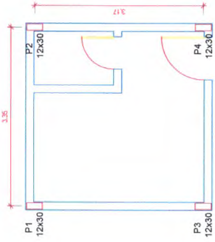
02 FORMAS PILARES Esc.: 1/50
