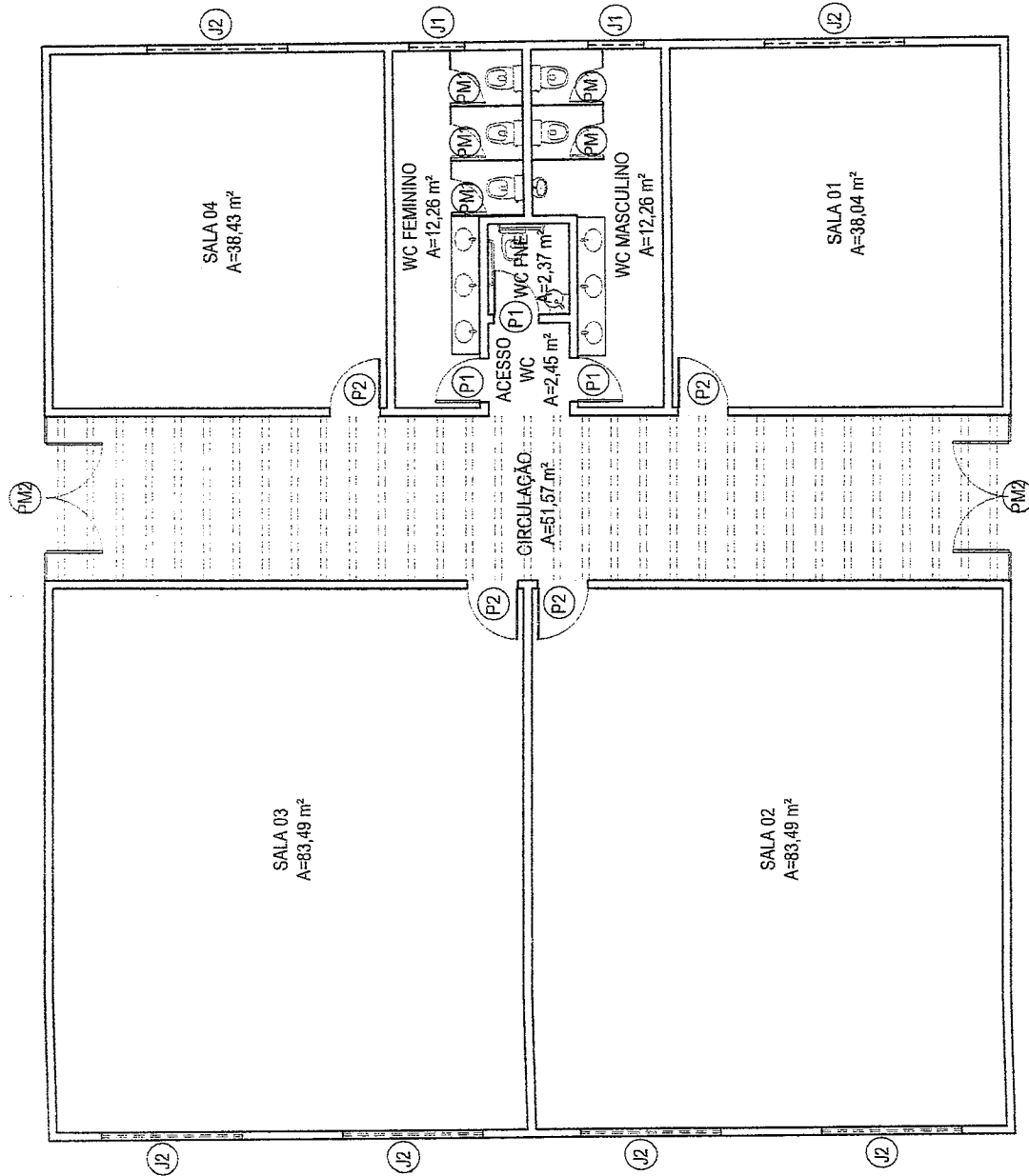
1 PLANTA BLOCO SALAS ESCALA 1:125
