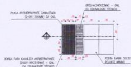
01 DETALHE A - PLANTA BAIXA
