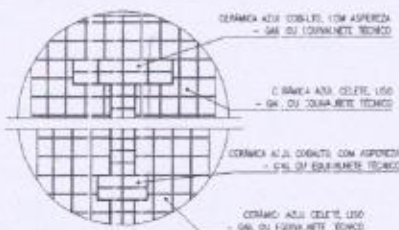
05 DETALHE D - PLANTA BAIXA
