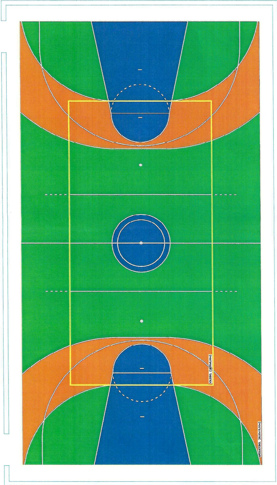
1 PLANTA BAIXA - PINTURA DA QUADRA ESCALA: 1/100
