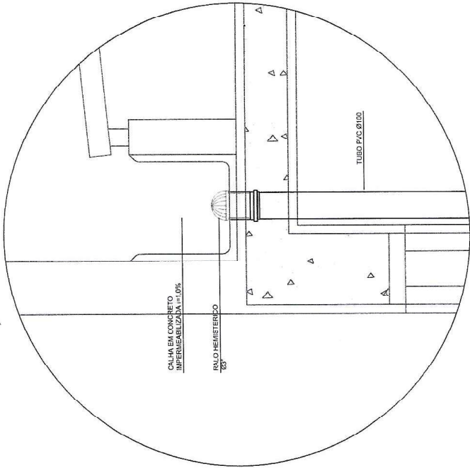
5 DETALHE - AMPLIAÇÃO CALHA ESC. S/E
