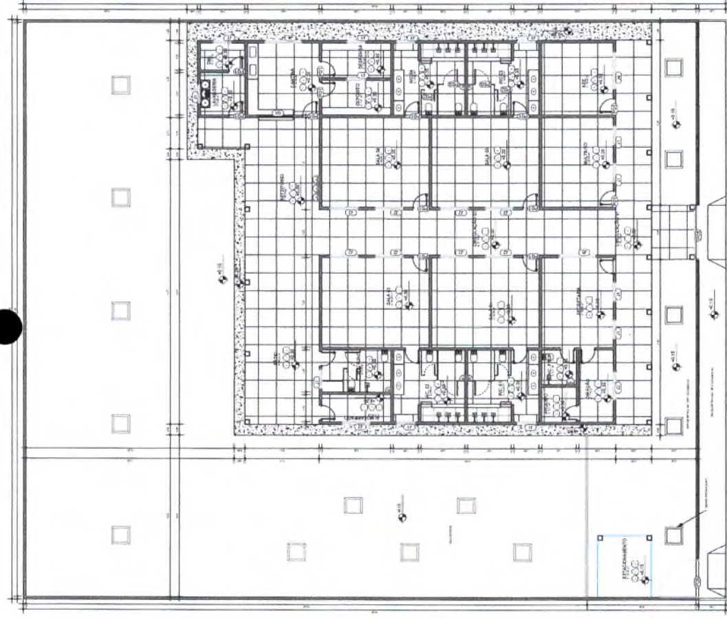
1 TÉRREO ESCALA - 1 : 100
